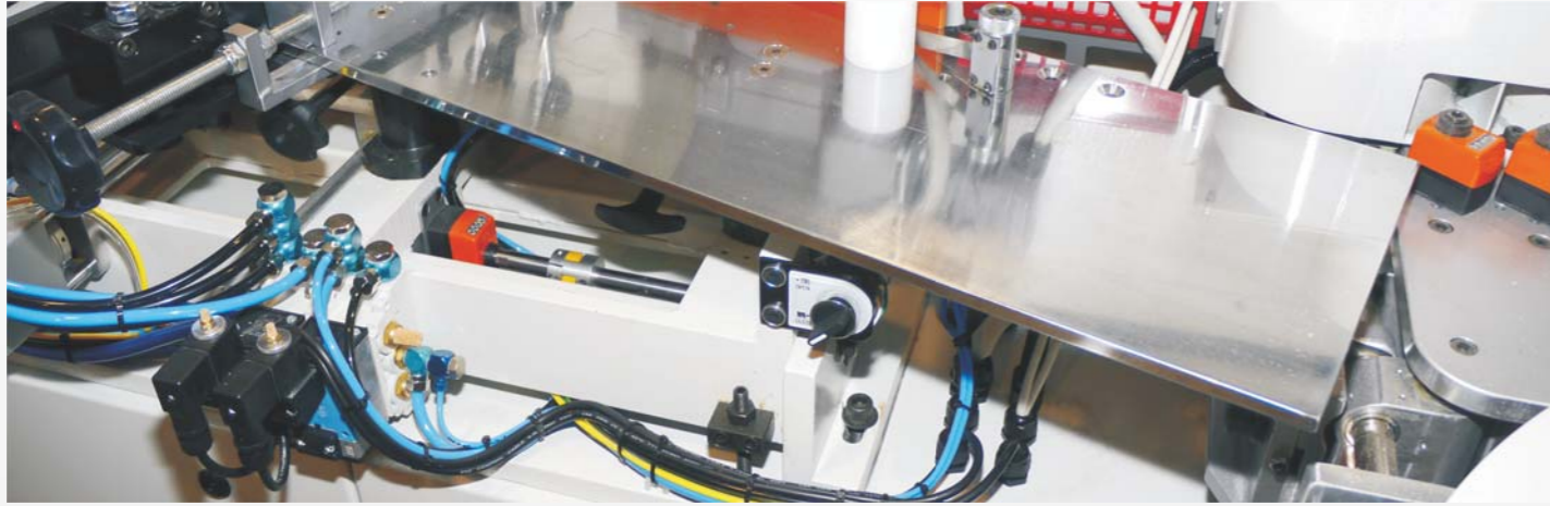
11. Height adjustable for infeed table 進料桌面高低微調裝置
