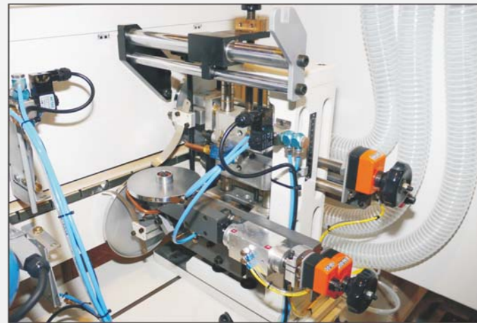
18. Profile scraping unit 型刮刀單元
