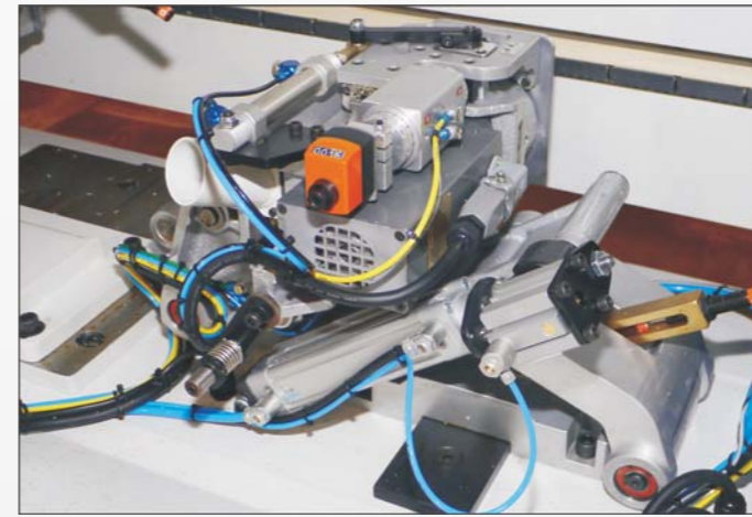
16. Multifunction contour copy unit 多功能仿角單元
