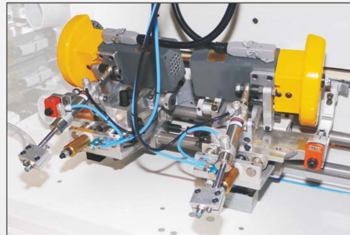
14. Compact tracking type snipping unit 精緻型水平前後修單元
