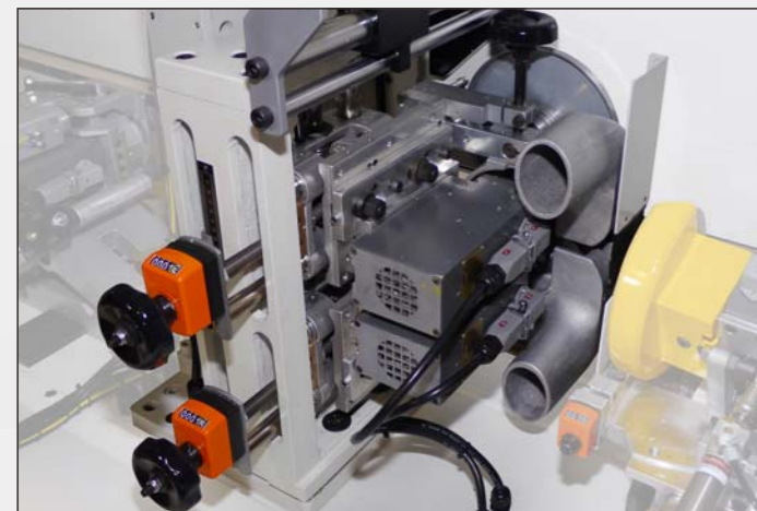
15. Rough trimming unit 上下修單元
