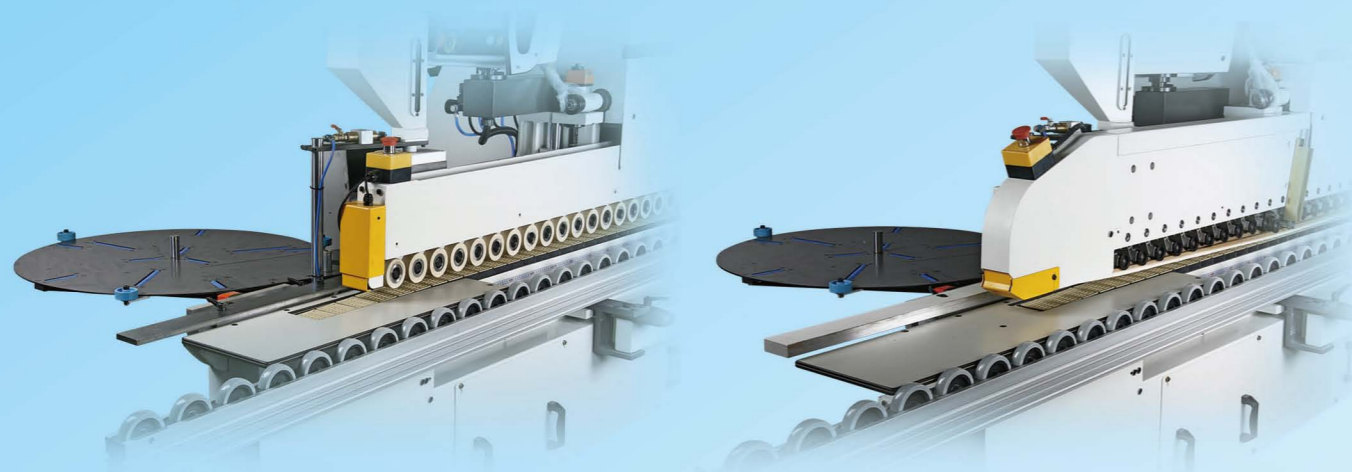
Left picture shown ROLLER TYPE for EB-2, EB-3. 左圖展示膠輪壓力樑。
